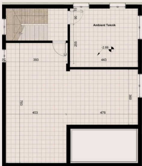
KATI NËNTOKË
